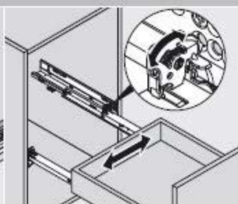
Compensation réglage latéral via coulisse arrière droite
